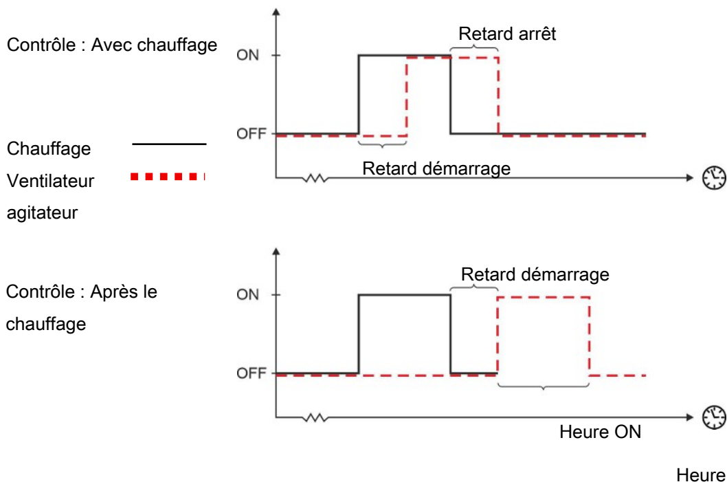
Figure 28: Contrôle avec chauffage
