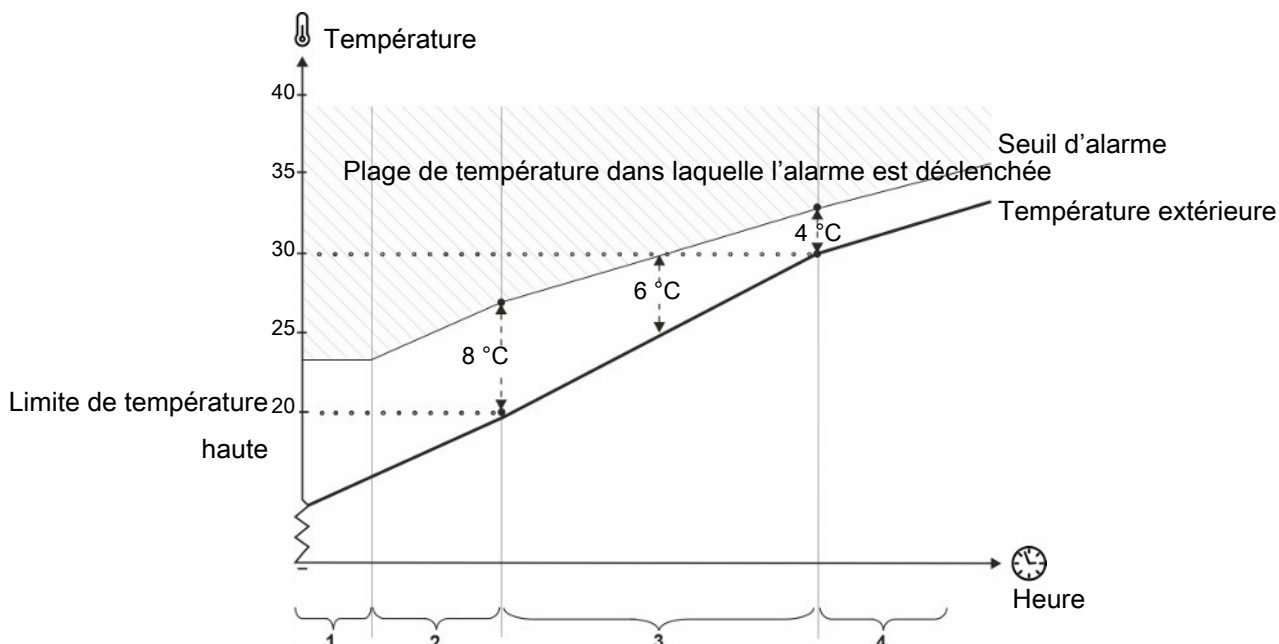
Figure 43: Température estivale à 20 °C et 30 °C à l'extérieur
