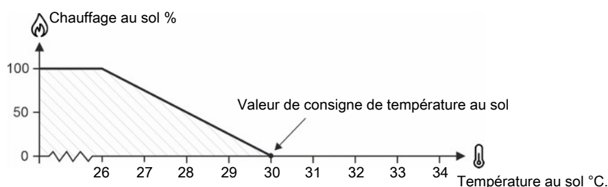
Figure 38: Chauffage au sol avec capteur thermique
