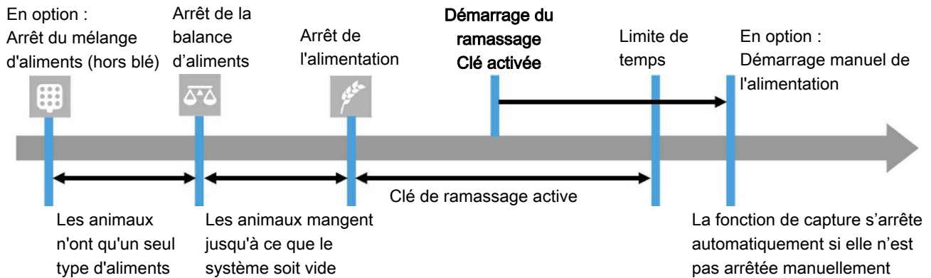
Figure 40: La séquence lors de l'arrêt du système d'alimentation pendant le ramassage
