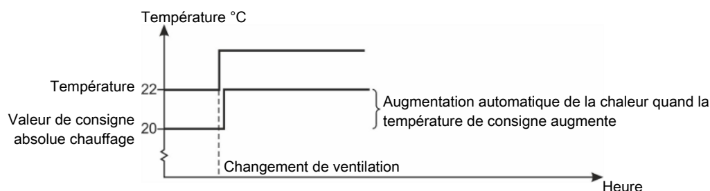
Figure 36: Alimentation en chaleur
