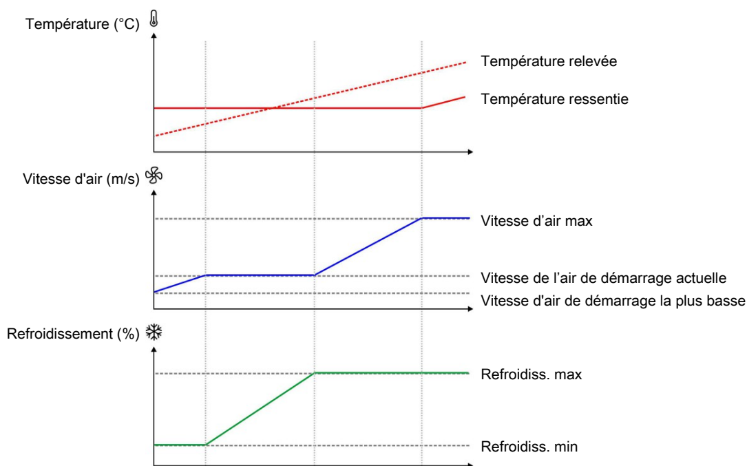
Figure 34: Le refroidissement démarre déjà à une vitesse d'air basse afin de maintenir la température intérieure requise. Lorsque le refroidissement ne parvient pas à maintenir la température, la vitesse d'air est de nouveau augmentée.
