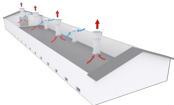
Figure 21: La ventilation FreeRange dans un système de pression égale
