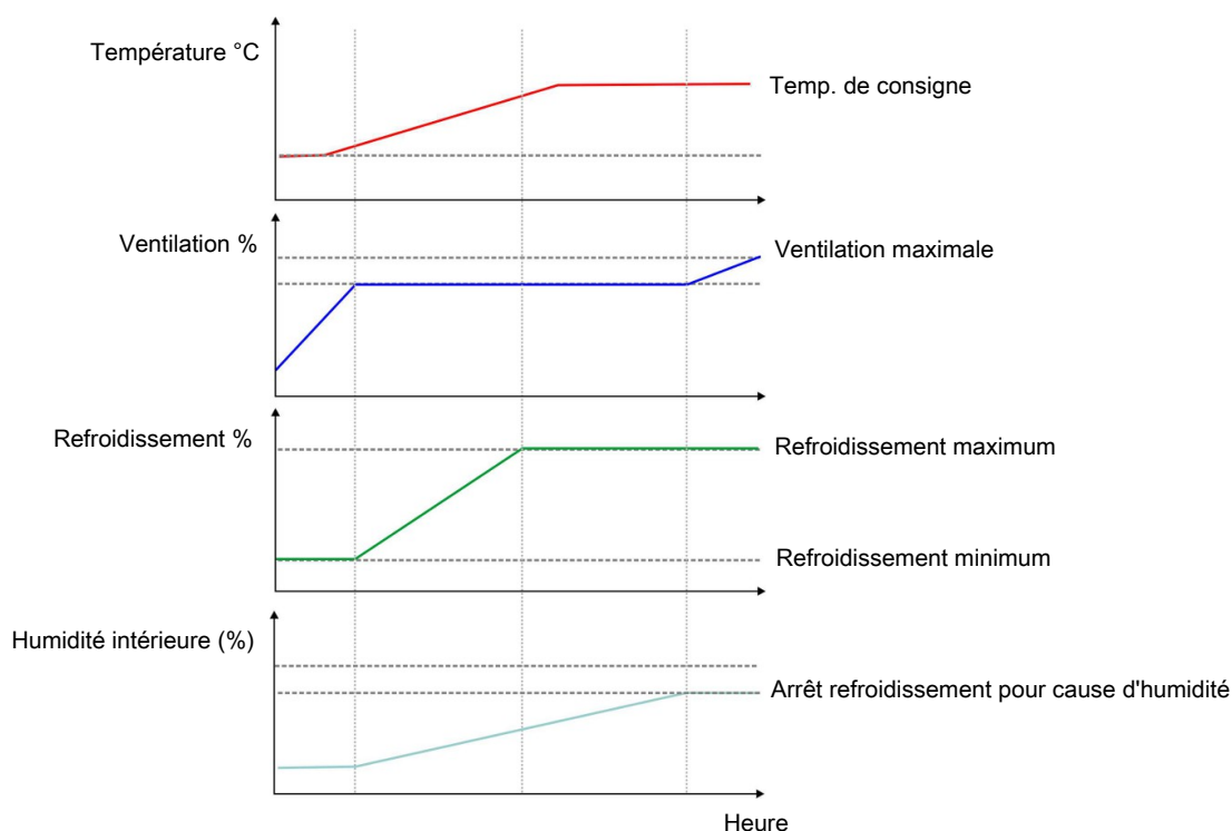
Figure 31: Pour maintenir la température intérieure requise, le refroidissement démarre avant que le niveau de ventilation n'ait atteint la ventilation maximale. Lorsque le refroidissement ne peut plus maintenir la température, la ventilation est augmentée à nouveau.
