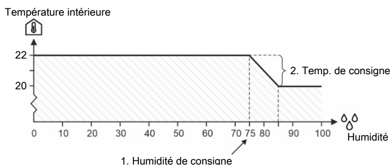
Figure 13: Contrôle de l'humidité avec réduction de température
