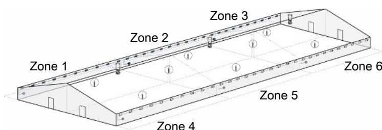
Figure 15: Exemple de bâtiment avec des entrées d'air contrôlées par zones.
