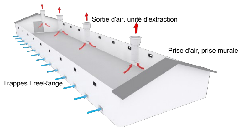
Figure 20: La ventilation FreeRange dans un système de pression négative
