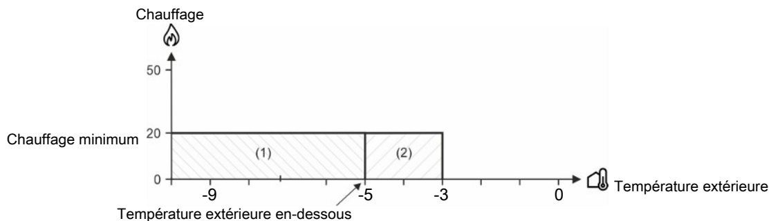
Figure 37: Chauffage minimum en cas de diminution ou d'augmentation de la température extérieure
