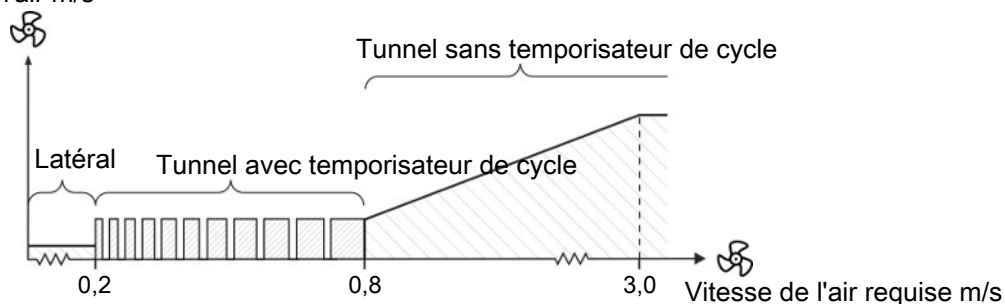
Figure 19: Séquence de ventilation avec temporisateur de cycle en ventilation mode tunnel
