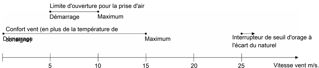
Figure 26: Ventilation naturelle à des vitesses du vent en augmentation
