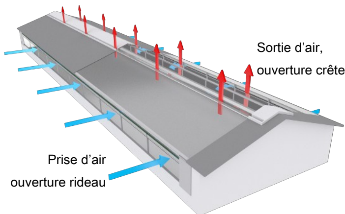
Figure 22: Par exemple, dans un bâtiment à la ventilation naturelle pure avec des ouvertures rideaux sur les côtés du bâtiment et une ouverture crête sur le toit.
