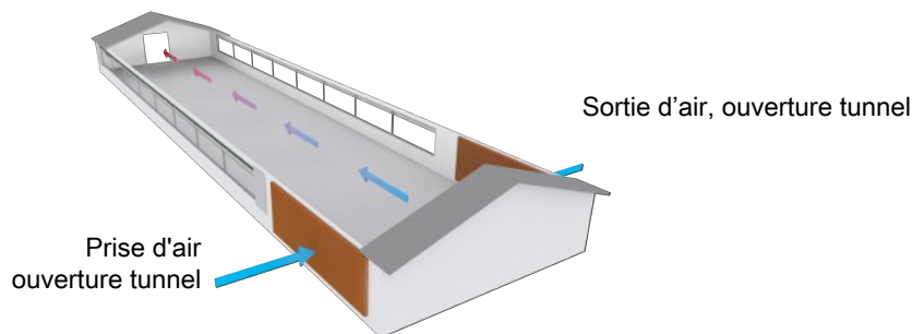
Figure 24: Exemple de bâtiment d'élevage à ventilation naturelle combiné à une ventilation tunnel, Ventilation tunnel.
