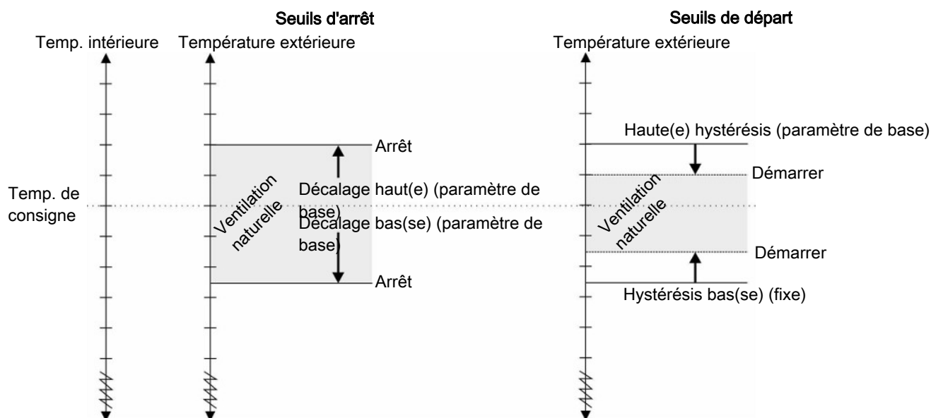
Figure 25: Démarrer et arrêter en fonction de la température extérieure. Les seuils de température sont définis comme étant décalés par rapport à la température de consigne.
